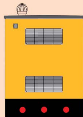
VISTA LATERALE DX
